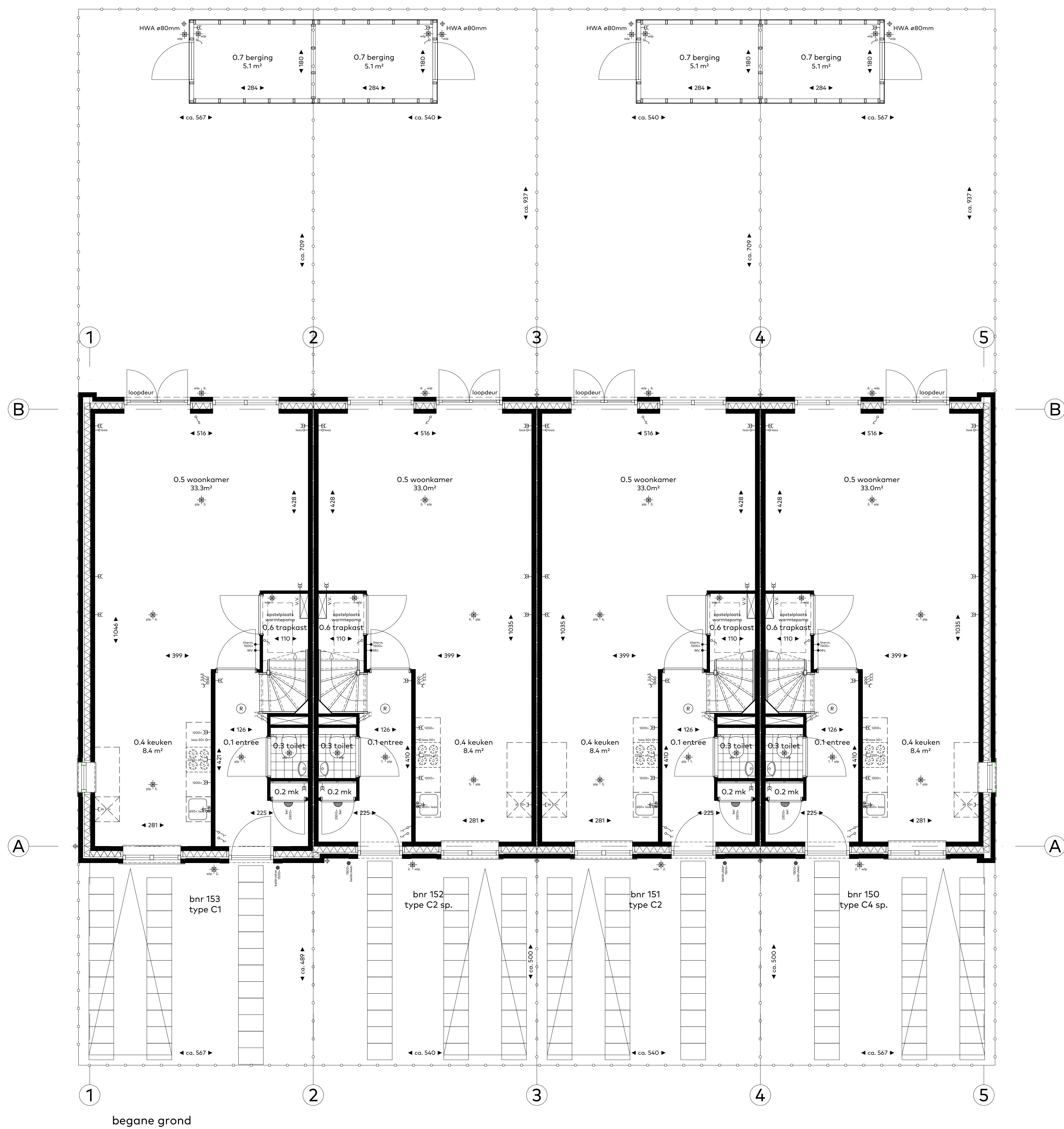
begane grond
