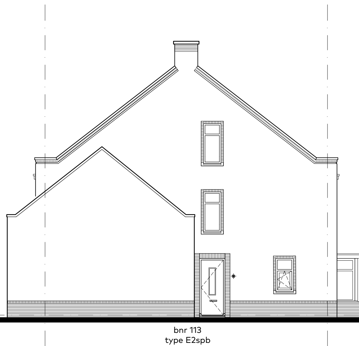
linkerzijgevel
