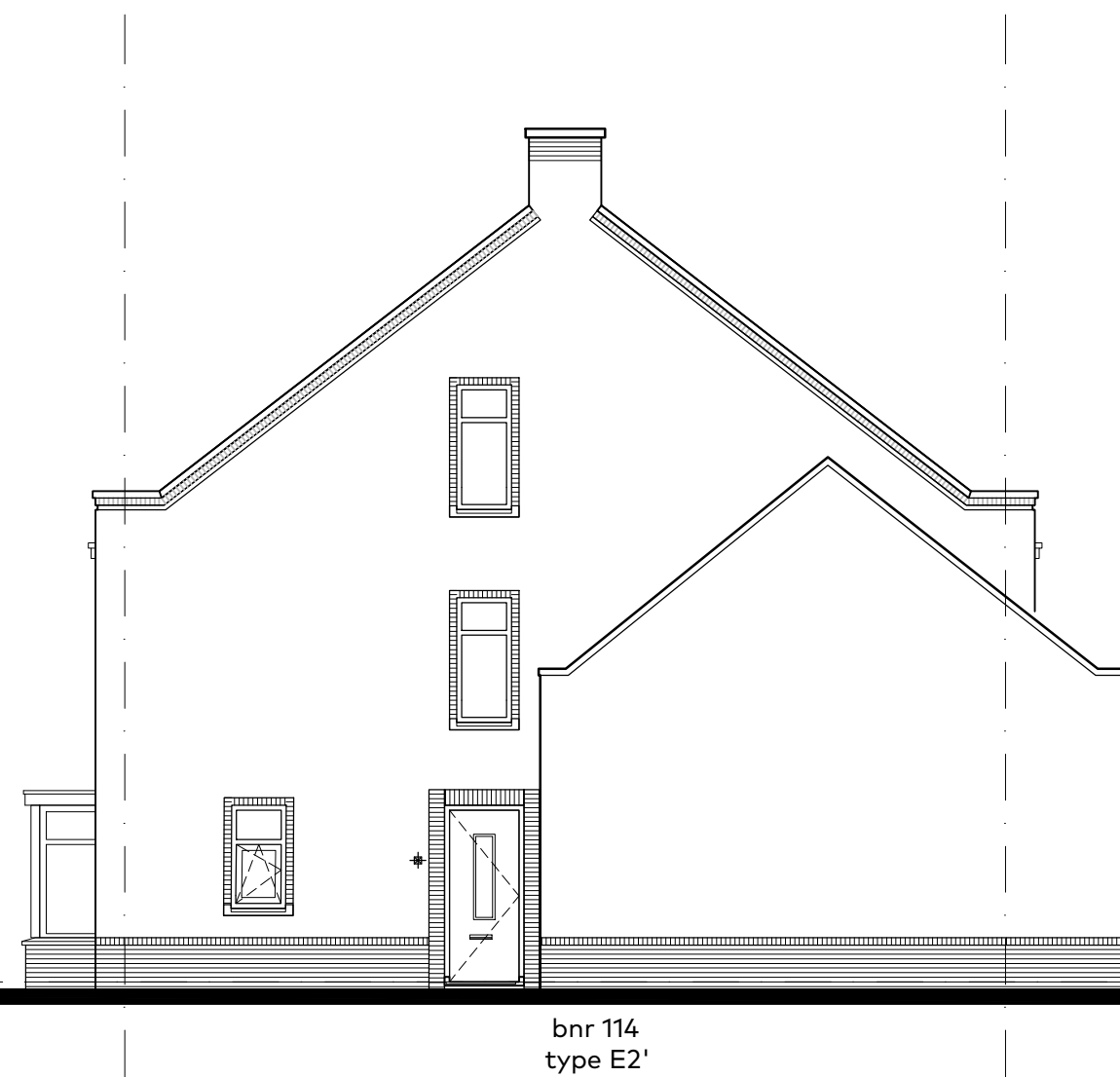
rechterzijgevel
