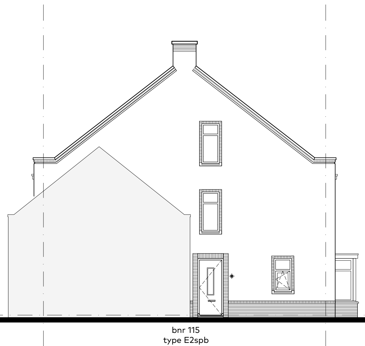
linkerzijgevel
